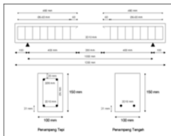
Gambar1. Penampang Memanjang dan Melintang Balok.
