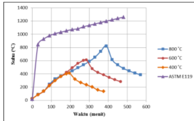
Gambar4. Kurva kenaikan dan penurunan suhu pembakaran
