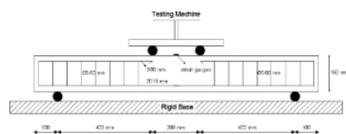
Gambar2. Setting Up Pengujian Lentur Balok dengan 2 Beban P
