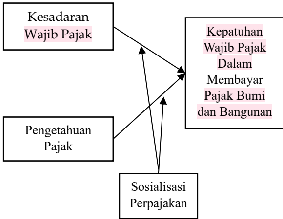
Gambar 1. Kerangka Konseptual
