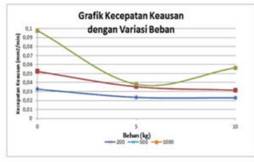
Gambar 6 Grafik kecepatan Keausan dengan Variasi Beban.
