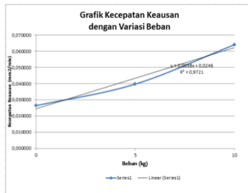
Gambar 7 Grafik Kecepatan Keausan dengan Variasi Beban.
