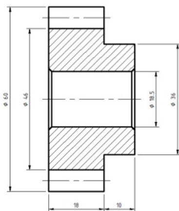
Gambar 4 Dimensi Roda Gigi
