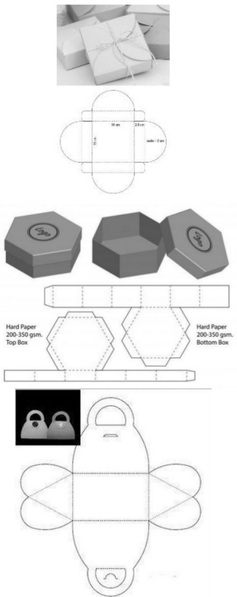
Gambar 3: Desain Gift Box
