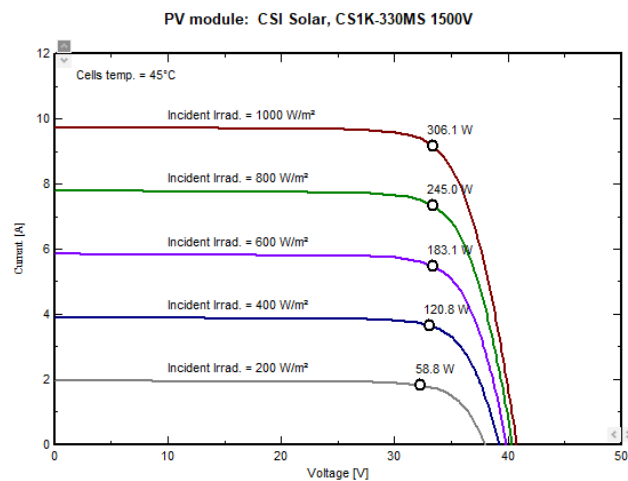
Gambar 3. Karakteristik Efek Si-Mono 330W, 30 V
