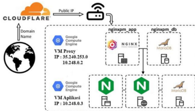
Gambar 2. Topologi Arsitektur Sistem
