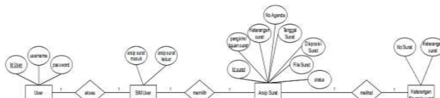
Gambar 9. ERD alur sistem informasi manajemen pengarsipan surat KPU Kota Malang untuk hak akses user
