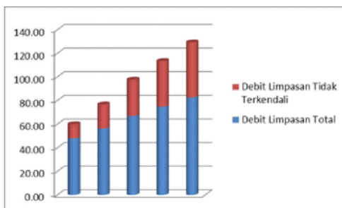
Gambar 7. Perbandingan Debit Limpasan Total dan Debit Limpasan Tidak Terkendali
