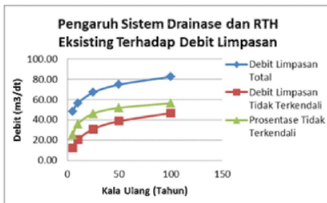
Gambar 6. Pengaruh Sistem Drainase dan RTH eksisting dalam penurunan debit limpasan pada daerah studi.
