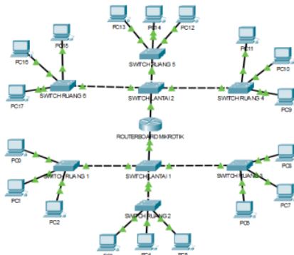
Gambar 2. Desain Topologi Jaringan
