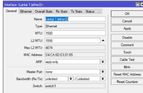
Gambar 11. Tampilan Penggantian Parameter ARP List
