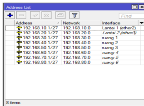
Gambar 3. Tampilan Address List Pada Winbox
