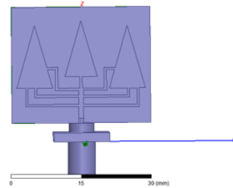
Gambar 6. Antena tampak depan
