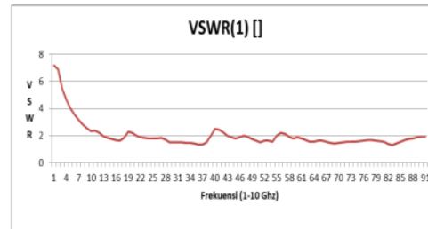
Gambar 9. Grafik nilai VSWR
