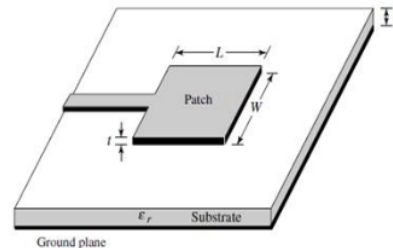
Gambar 1 Bagian-bagian Antena Mikrostrip
