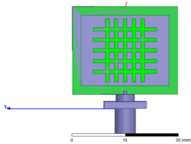
Gambar 7. Antena tampak belakang
