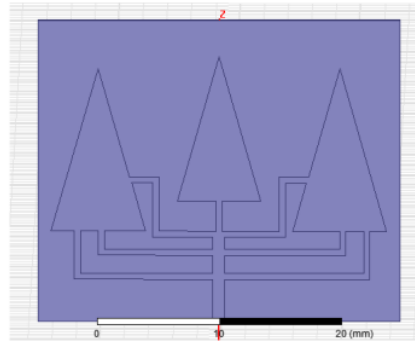
Gambar 4. Substrat dan Patch
