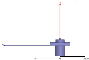
Gambar 2 Pembuatan Port
