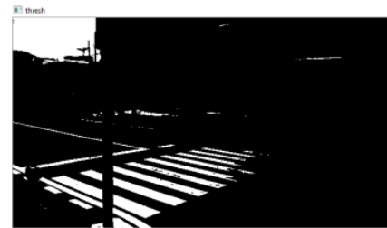
Gambar 6. threshold terbaik 180
