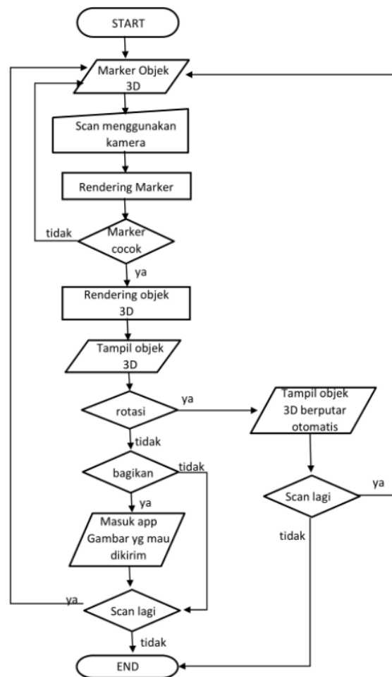
Gambar 2. Diagram Alir Aplikasi Buwung AR
