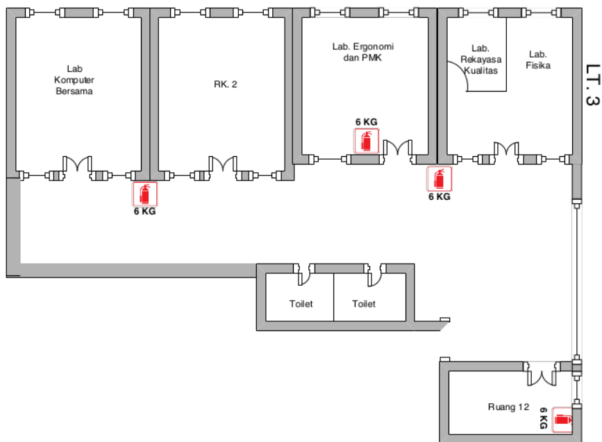
Gambar 3 . Rancangan Usulan Penempatan APAR pada Lantai 3 Gedung Laboratorium
