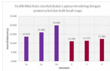
Gambar 5. Grafik nilai ketebalan lapisan anodizing dengan pewarna kol dan kulit buah naga
