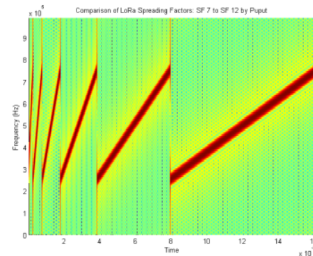
Fig. 6. Comparison Spreading Factor (SF) pada 500 kHz Frequency.
