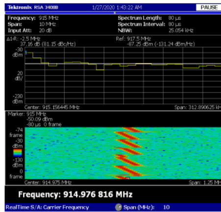
Fig. 29. LoRa Chirp Signal.
