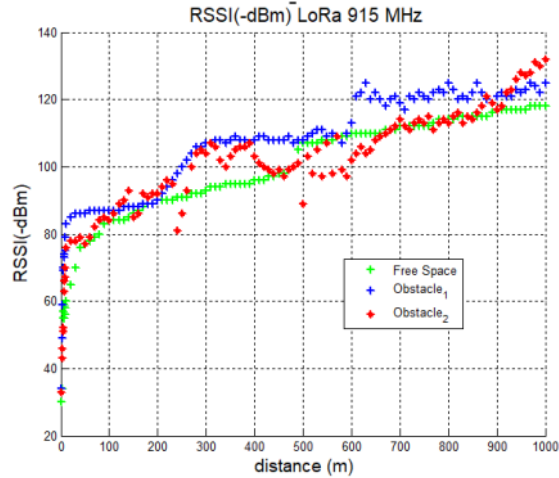
Fig. 23. RSSI (-dBm) LoRa 915 MHz.
