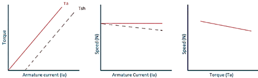
Gambar 3.4 Grafik Karakteristik Motor DC Shunt – Torsi vs Arus Jangkar,
