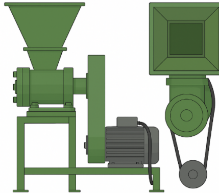
Gambar 2.40. Ilustrasi struktur rangka mesin cetak pakan tampak samping dan tampak atas menunjukkan pemilihan material dan sambungan rangka.
