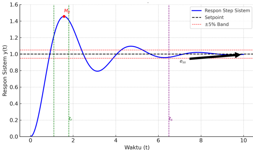
Gambar 5.1 Ilustrasi parameter kinerja sistem kontrol.
