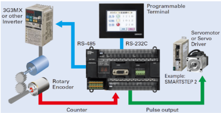
Gambar 5.12 Ilustrasi skema sistem kontrol berbasis PLC dengan fungsi komunikasi dan pulsa I/O.
