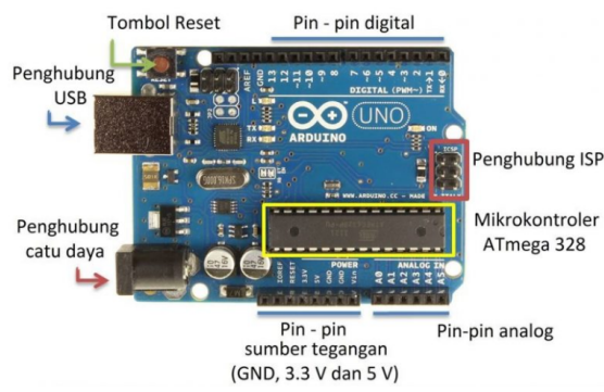
Gambar 5.9 Tampilan Arduino Uno dan bagian-bagiannya.
