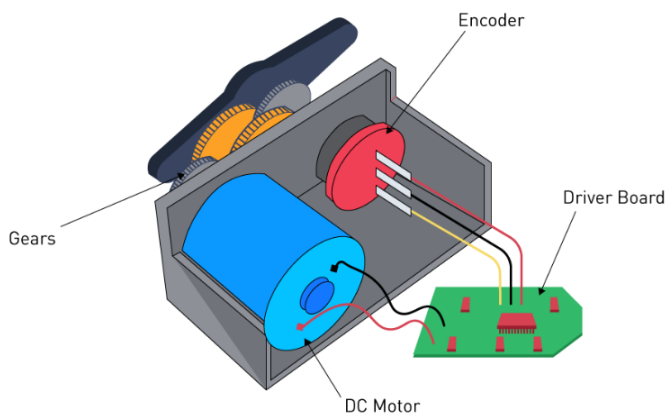
Gambar 3.13 Komponen Motor Servo.
