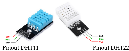
Gambar 4.5 Sensor kelembapan DHT11 dan DHT22.
