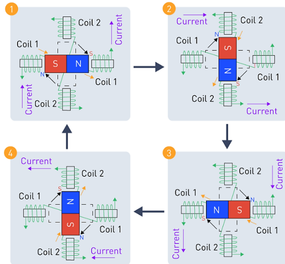
Gambar 3.11 Prinsip dasar pengoperasian motor stepper (Bianculli, 2009).
