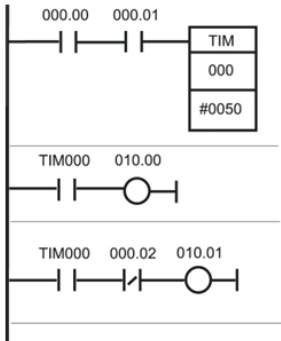
Gambar 5.13 Contoh diagram tangga PLC: 000.xx/010.xx—grup alamat input/output, TIM000—penundaan timer 5 detik. 000.00—kontak input normal terbuka, 000.02—kontak input normal tertutup.
