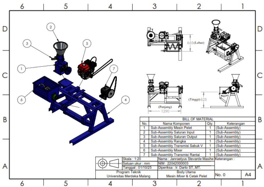
Gambar 6.4 Ilustrasi skematik desain mesin pellet.
