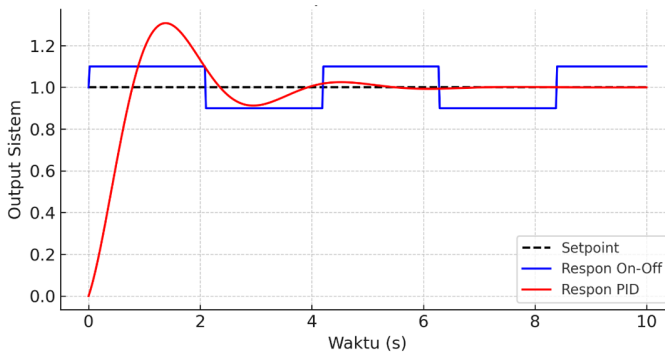
Gambar 5.5 Ilustrasi skema respon sistem kontrol On-Off vs PID.
