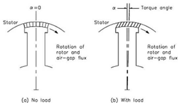
Gambar 3.7 Sudut Torsi
