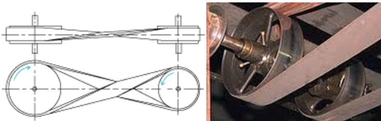
Gambar 2.16 Konstruksi sabuk rata silang ( cross flat belt ).
