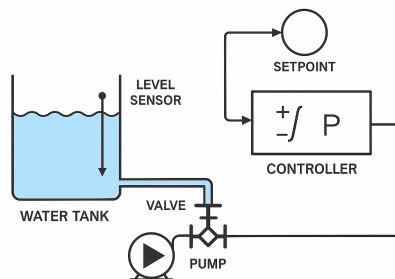
Gambar 4.2 Ilustrasi Diagram Sistem Kendali Level Fluida.
