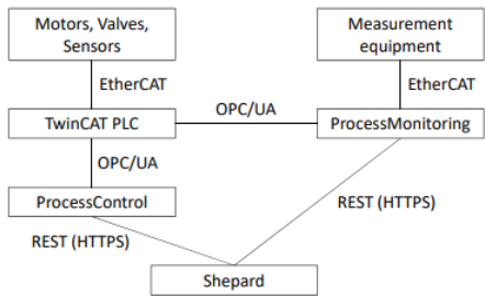
Gambar 4.13 Ilustrasi skematik sistem akuisisi data terintegrasi dengan PC dalam proses pengelasan.
