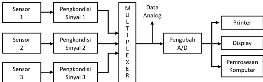
Gambar 4.18 Ilustrasi skema blok diagram sistem akuisisi data.
