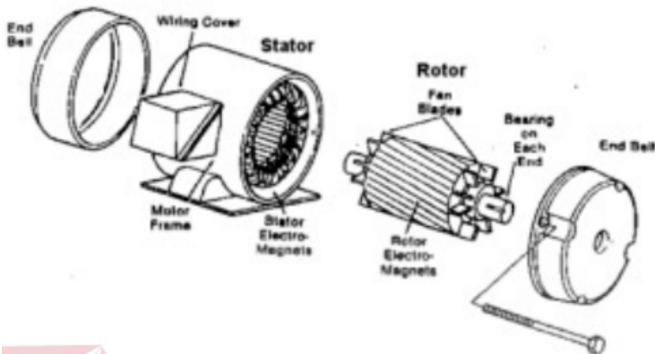
Gambar 3.8 Konstruksi Motor AC Asynchron (Aripriharta, 2023)
