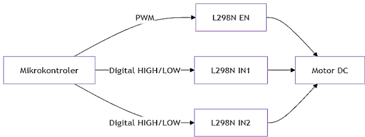
Gambar 3.15 Diagram driver dasar motor DC dengan H-Bridge (L298N).
