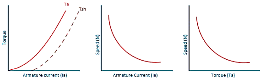
Gambar 3.3 Ilustrasi grafik karakteristik motor DC Seri – Torsi vs Arus Jangkar, Kecepatan vs Arus Jangkar, Kecepatan vs Torsi.
