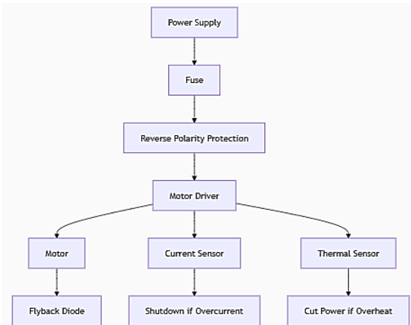
Gambar 3.17 Contoh diagram rangkaian proteksi.
