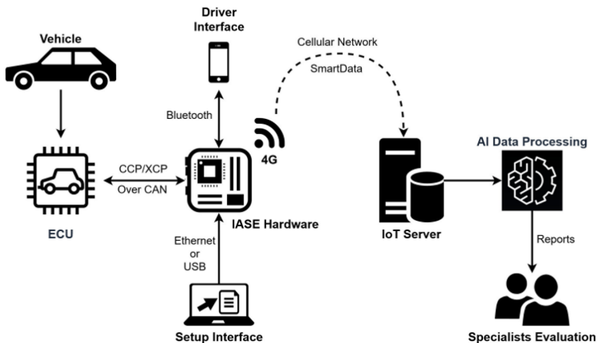
Gambar 4.19 Ilustrasi sistem skuisisi data mandiri pada unit kendali elektronik otomotif.
