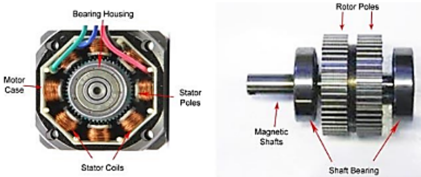
Gambar 3.10 Konstruksi Motor Stepper, a. Stator, b. Rotor.
