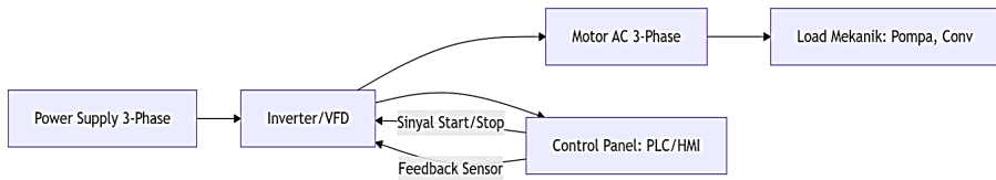
Gambar 3.18 Diagram Sistem Kelistrikan dengan Inverter
