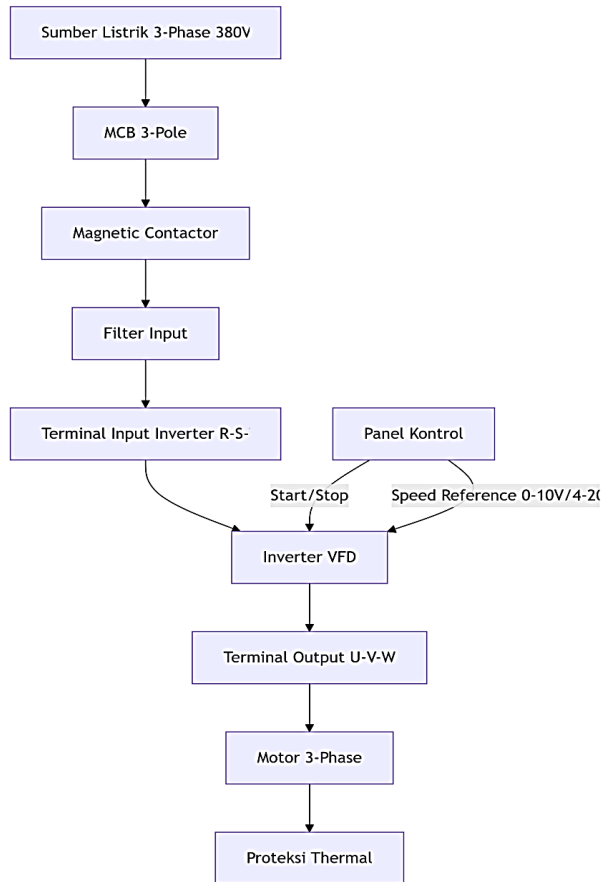
Gambar 3.19 Diagram Blok Sistem Pengendalian Motor 3-Phase dengan Inverter (VFD).
