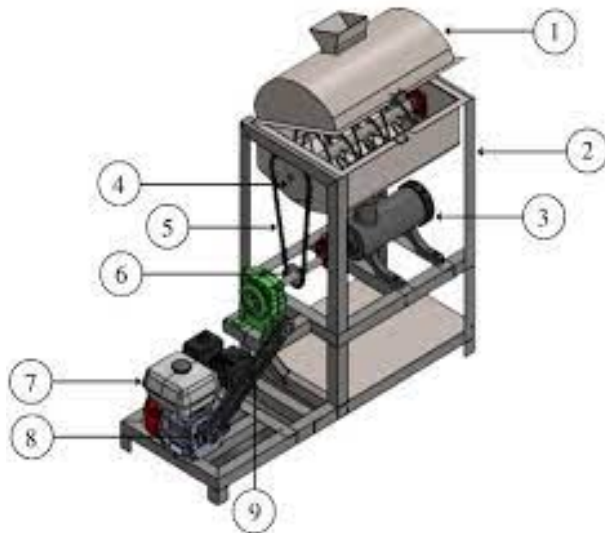
Gambar 2.38 Ilustrasi diagram sistem screw conveyor dan extruder pada mesin cetak pakan. Bagian-bagiannya:
