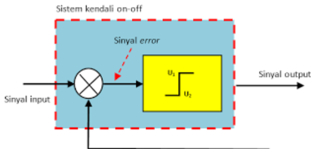
Gambar 5.2 Ilustrasi diagram blok sistem kontrol On-Off .
