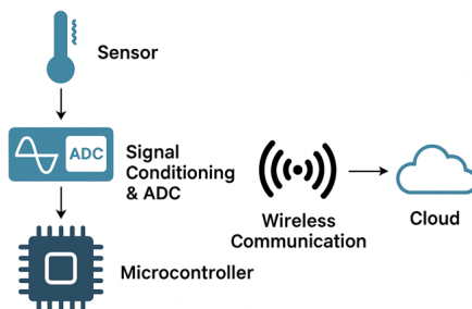
Gambar 4.15 Ilustrasi diagram sistem akuisisi data wireless (Nirkabel).
