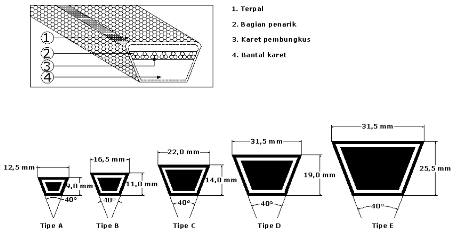
Gambar 2.13 Tipe dan ukuran sabuk V.
