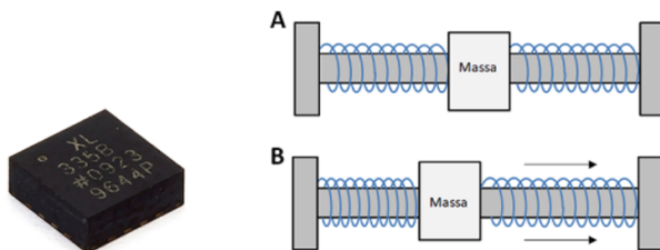
Gambar 4.10 Bentuk chip sensor akselerometer dan prinsip kerjanya.
