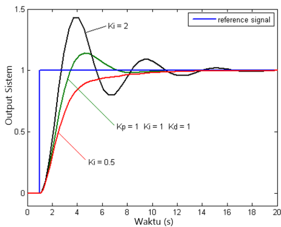
Gambar 5.4 Ilustrasi kurva Y vs waktu, untuk tiga nilai K_p ( K_i dan K_d dijaga konstan).
