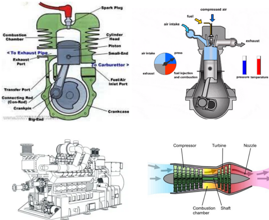
Gambar 2.1 Mesin pembakaran dalam.
