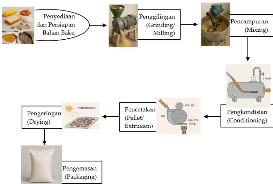
Gambar 6.1 Ilustrasi skematik aliran proses mesin cetak pakan otomatis.
