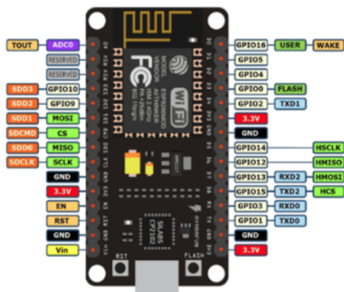
Gambar 5.10 NodeMCU ESP8266.
