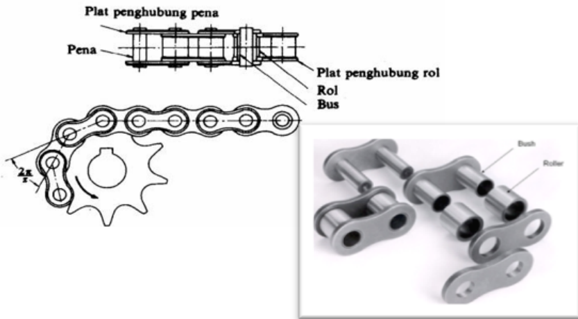
Gambar 2.18 Komponen rantai transmisi.
