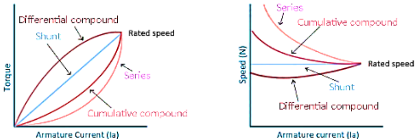
Gambar 3.5 Grafik Karakteristik Motor DC Coumpound kumulatif dan Coumpound diferensial.
