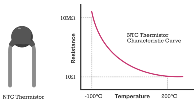
Gambar 4.4 Sensor suhu dan karakteristik kurvenya.
