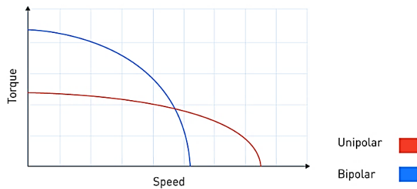
Gambar 3.12 Perbandingan karakteristik Kecepatan-Torsi pada motor stepper.
