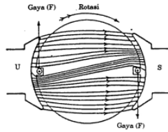
Gambar 3.2c Interaksi kedua medan magnet dalam menghasilkan gaya.
