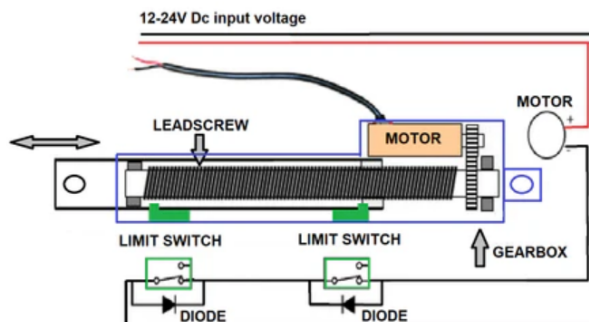
Gambar 1.3 Rangkaian aktuator linier elektrik dengan motor DC, leadscrew , gear box , dan limit switch .
