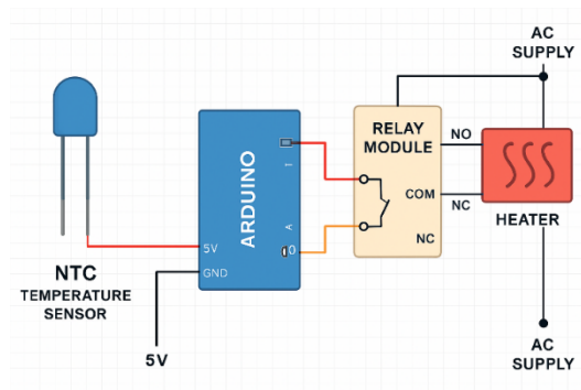
Gambar 5.15 Ilustrasi diagram wiring sistem kontrol suhu.
