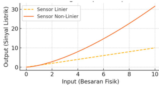
Gambar 4.3 Ilustrasi Grafik hubungan input-output antara sensor linier dan non-linier.
