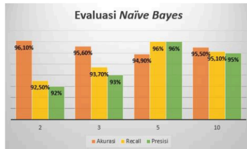
Gambar 2. Evaluasi Naive Bayes dengan Cross-Validation
