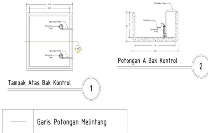
Gambar 6. Detail Rumah Pompa Atau bak Kontrol
