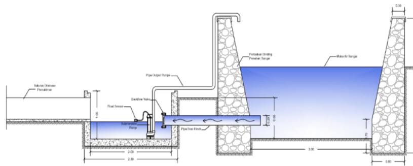
Stasiun Pompa Kondisi Dua
