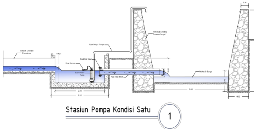
Gambar 7. Gambar pompa pada kondisi Satu
