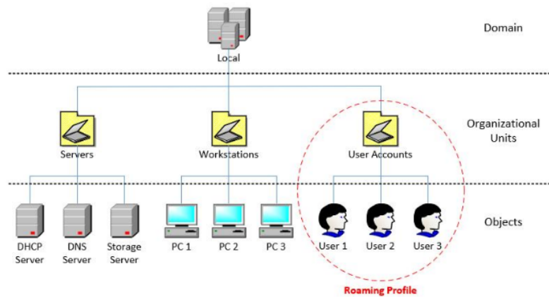
Gambar 5. Struktur Organizational Unit (OU)
