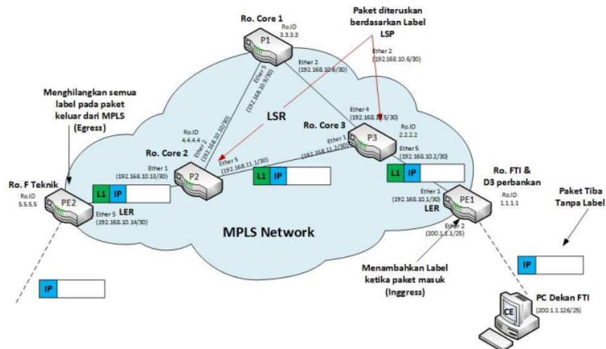
Gambar 7 Informasi jalur label swiching path
