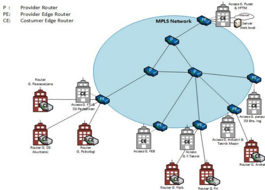
Gambar 1. Simulasi perancangan jaringan Universitas Merdeka Malang
