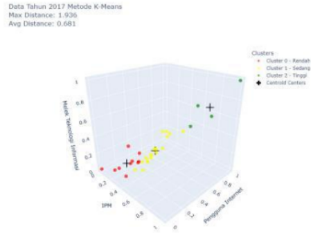
Gambar 8. Grafik 3D Scatter Plot hasil dari K-Means klustering data tahun 2017
