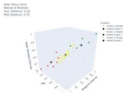
Gambar 13. Grafik 3D Scatter Plot hasil dari K-Medoids klustering tahun 2019
