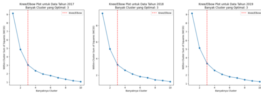
Gambar 7. Grafik Knee/Elbow data tahun 2017 hingga 2019
