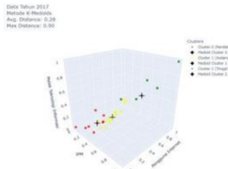
Gambar 12. Grafik 3D Scatter Plot hasil dari K-Medoids klustering tahun 2017
