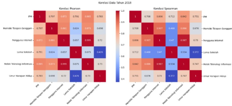
Gambar 6. Grafik Heatmap korelasi data tahun 2018
