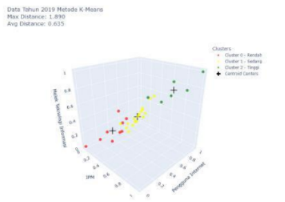
Gambar 9. Grafik 3D Scatter Plot hasil dari K-Means klustering data tahun 2019
