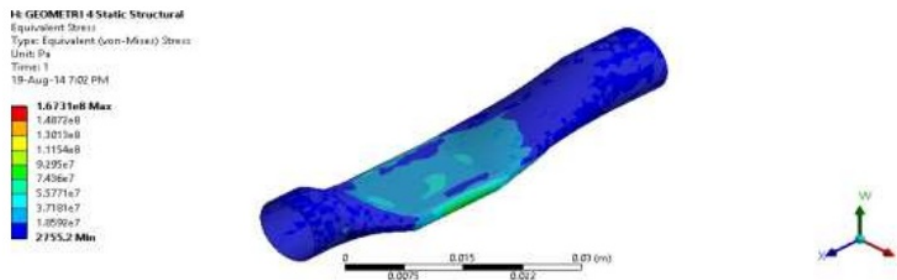
Gambar 13. Simulasi Tegangan Struktur Model Geometri-4
